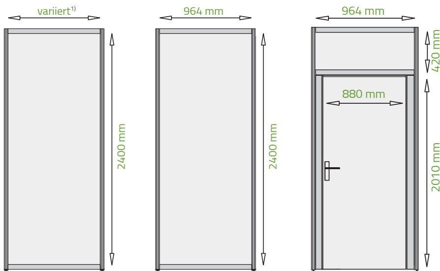
① Wand Sondermaß 1) ② Standardwand ③ Kabinentür und ④ Türsturz
