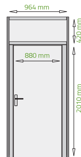
④ Kabinentür und ⑤ Türsturz
