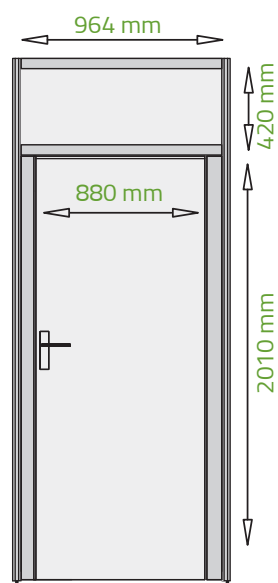
③ Kabinentür und ④ Türsturz
